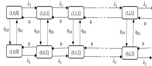
Figure 24.2. Le diagramme de transition de modèle RdPSG - MMPP/M/1 .
