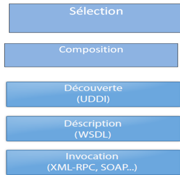
Figure 29.1. Web service - Modèle en couches.
