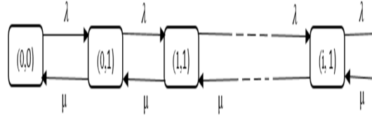
Figure 24.5. Le diagramme de transition du modèle RdPSG - MMPP/M/1 .
