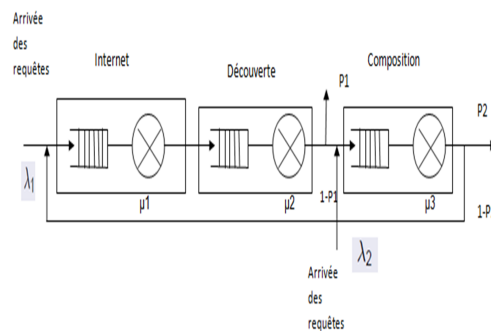
Figure 29.2. Modèle d'un système des Web services.
