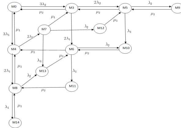
Figure 20.3. La CMTc associée au RdPSG de M_2/M_2/1//3 .
