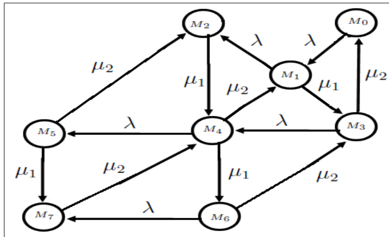
Figure 22.3. CTMC associé au GSPN (cas où N=2 ).
