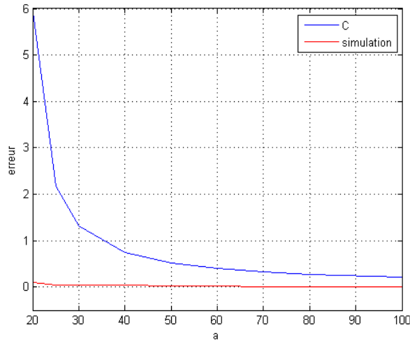
Figure 3.4. Courbes comparatives des erreurs.
