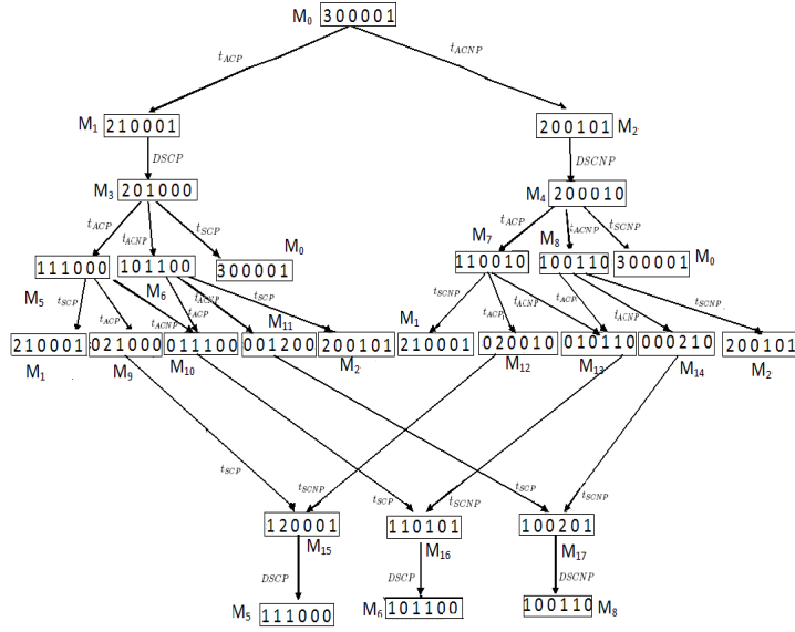
Figure 20.2. Graphe d'accessibilité associé au système M_2/M_2/1//N .
