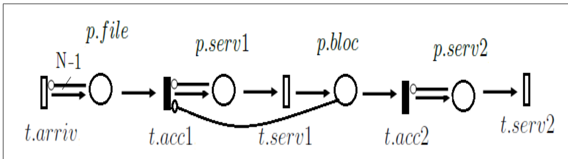
Figure 22.2. Le GSPN associé au M/M/1/N \rightarrow \bullet/M/1/1 .
