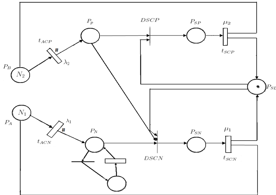
Figure 21.1. Le RdPSG modélisant les systèmes M_2/M_2/1/(N_1, N_2) avec rappels
