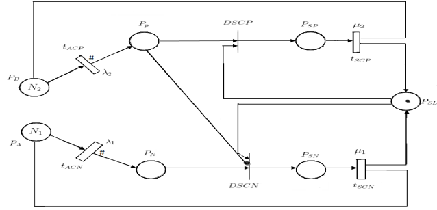
Figure 20.5. Le RdPSG modélisant les systèmes M_2/M_2/1/(N_1, N_2) avec priorité relative.
