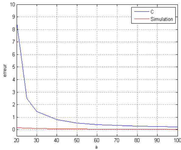
Figure 3.3. Courbes comparatives des erreurs.
