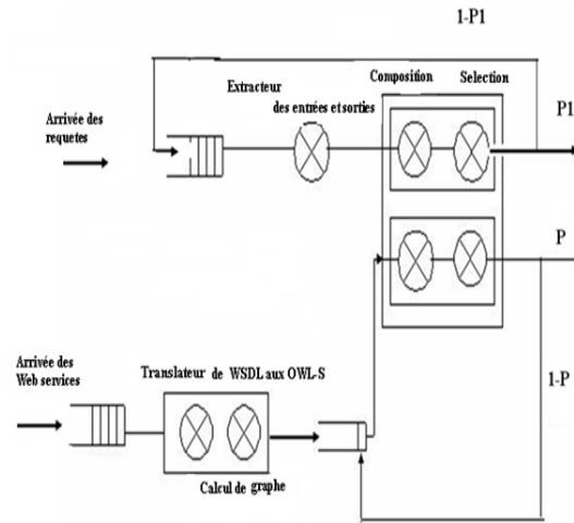
Figure 28.2. Modèle de composition des Web services par un graphe.
