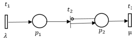
Figure 24.4. Le modèle RdPSG - M/M/1 .
