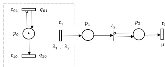
Figure 24.1. Le modèle RdPSG - MMPP/M/1 .
