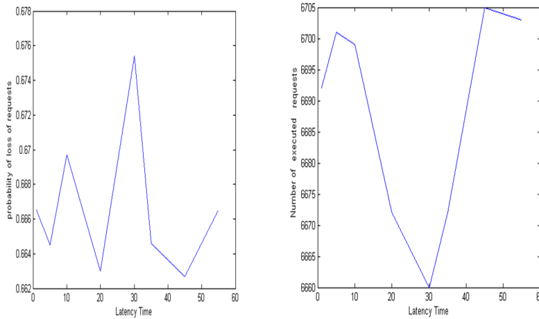
Figure 28.3. La probabilité de perte des requêtes et le nombre de requêtes exécutés en fonction du temps de latence.
