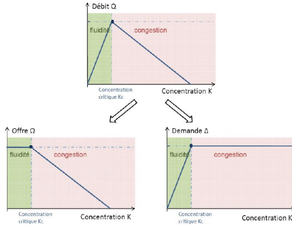
Figure 30.1. Diagramme fondamental triangulaire.
