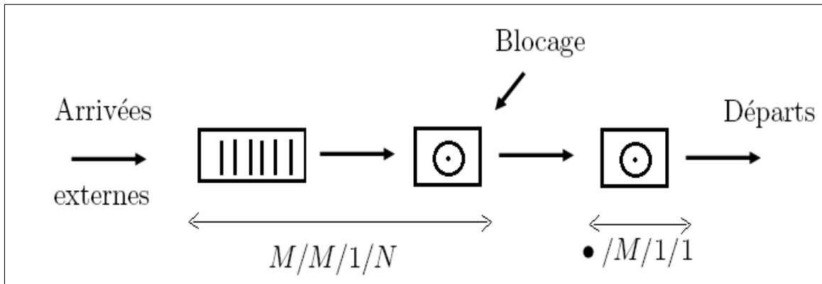
Figure 22.1. Le réseau M/M/1/N \rightarrow \bullet/M/1/1 .
