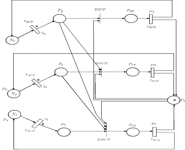
Figure 20.9. Le RdPSG modélisant le système M_3/M_3/1//((N_1, N_2, N_3) avec priorité relative.
