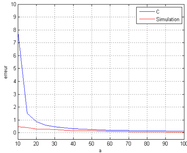
Figure 3.2. Courbes comparatives des erreurs.
