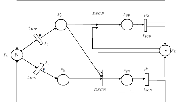
Figure 20.1. Le RdPSG modélisant les systèmes M_2/M_2/1//N avec priorité relative.
