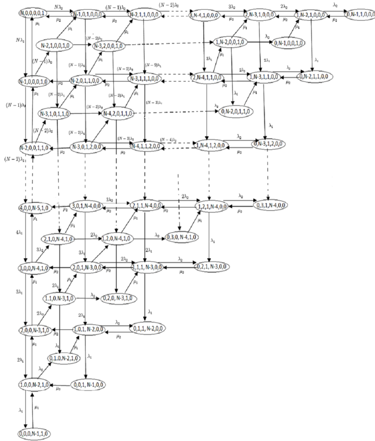
Figure 20.4. La CMTC associée au RdPSG de M_2/M_2/1//N .
