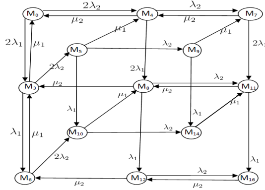
Figure 20.7. La Chaîne de Markov du réseau de Petri associé à M_2/M_2/1/(2, 2) avec priorité relative.
