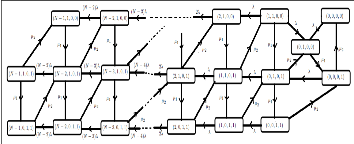
Figure 22.4. CTMC associé au GSPN (cas où N est quelconque).
