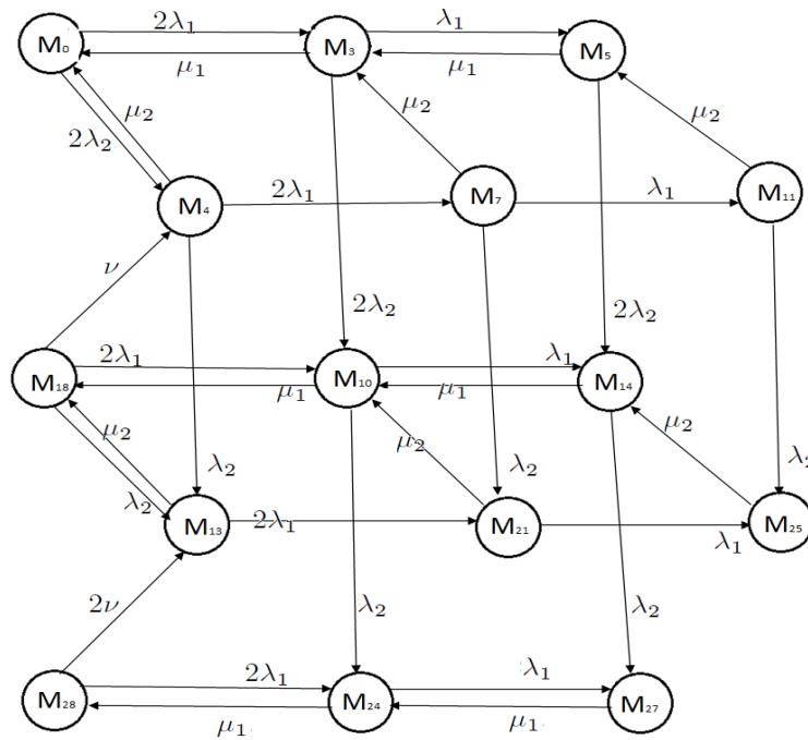
Figure 21.2. La CTMC pour les systèmes M_2/M_2/1//(\mathbf{2}, \mathbf{2}) avec rappels.
