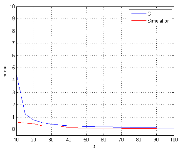
Figure 3.1. Courbes comparatives des erreurs.
