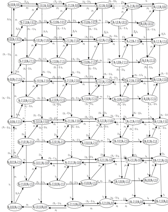
Figure 20.8. La CMTC associée à M_2/M_2/1/(N_1, N_2) .
