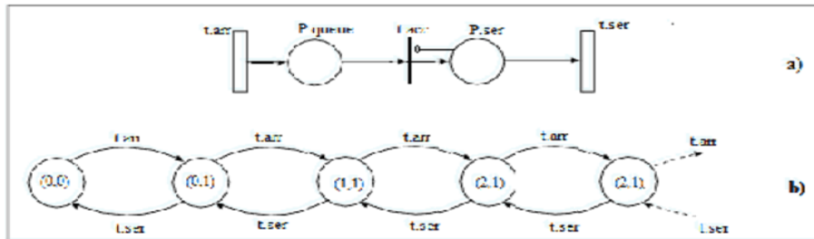
Figure 23.2. Le M/G/1 - MRSPN et son graphe d'accessibilité
