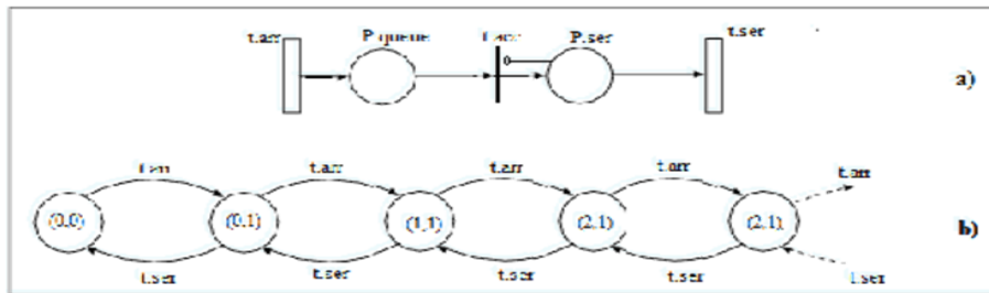
Figure 23.1. Le M/M/1 - GSPN et son graphe d'accessibilité
