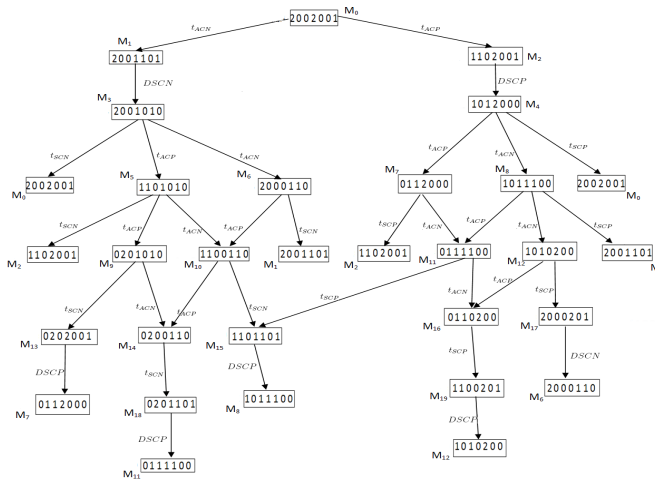
Figure 20.6. Graphe d'accessibilité associé à M_2/M_2/1/(2, 2) avec priorité relative.
