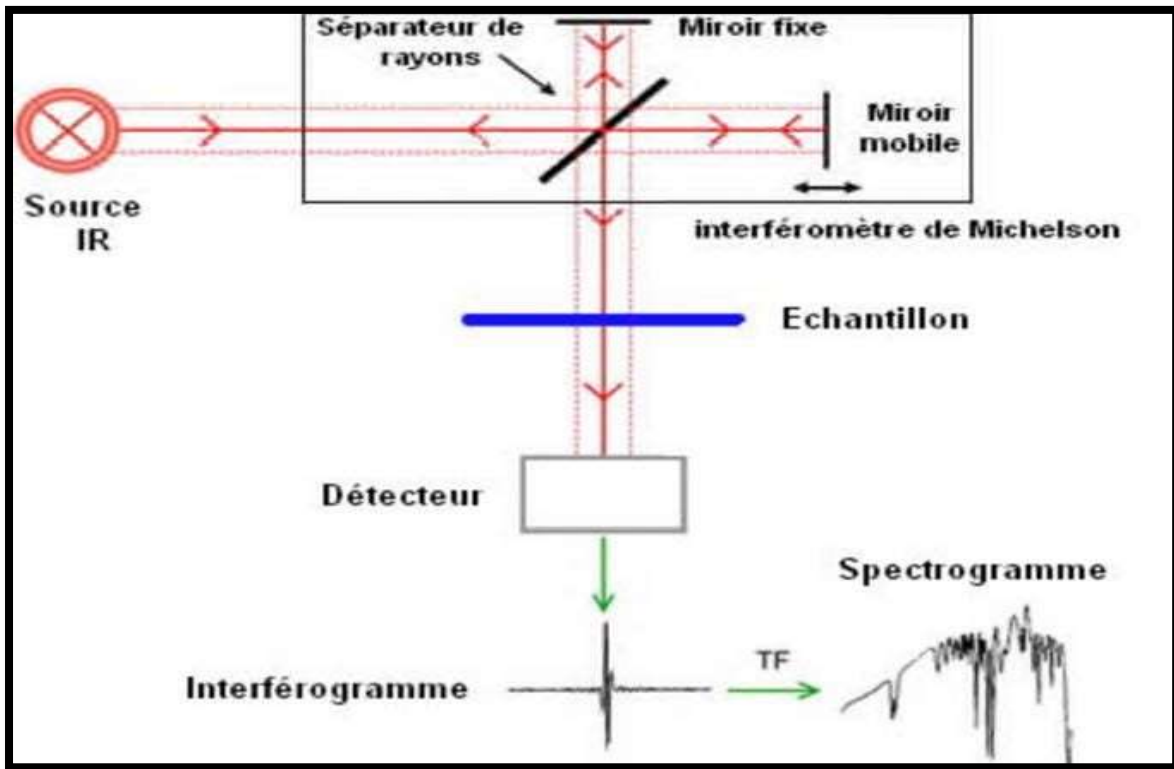
Figure II.10. Schéma de principe de l'analyse par spectroscopie d'absorption infrarouge [53]
