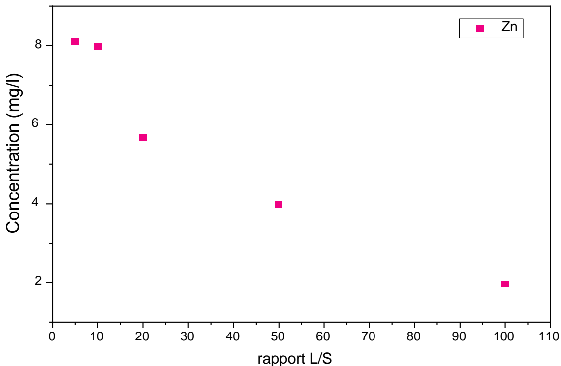
Figure III.11. Évolution de concentration du zinc selon les tests EP et FMM pour le matériau S/S.
