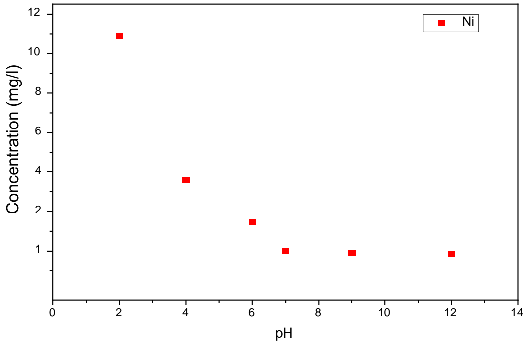
Figure III.7. Evolution de la concentration du nickel en fonction du pH pour le matériau S/S.
