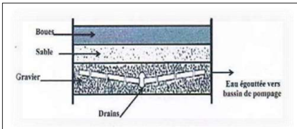
Figure II.2 : Coupe représentative de la composition d'un lit de séchage
