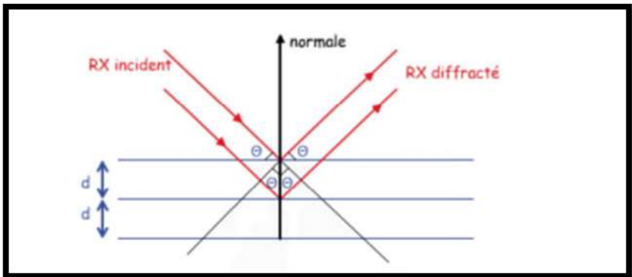
Figure II.7. Schéma de diffraction des rayons X par une famille de plan réticulaire. d est la Distance réticulaire, \theta est l'angle de Bragg [56]
