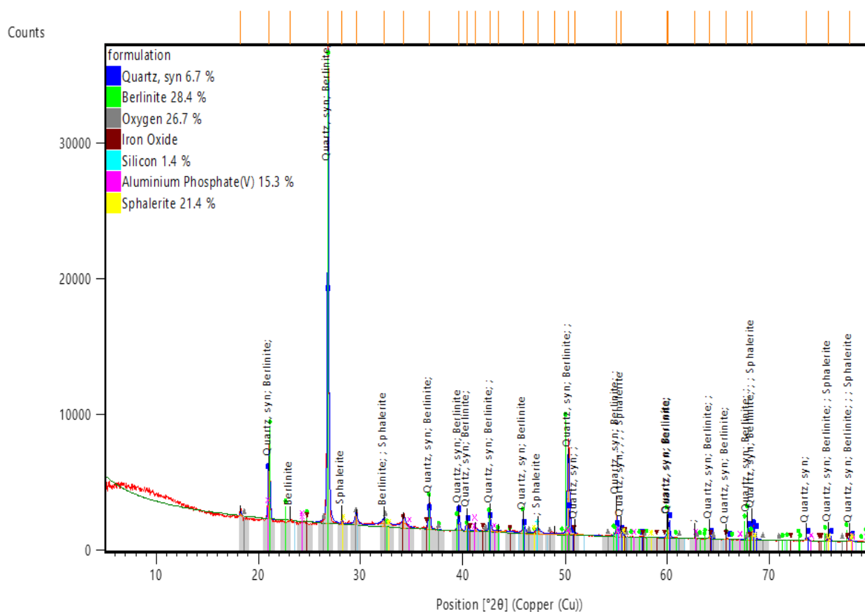
Figure III.3. Diffractogramme de la formulation analysée.
