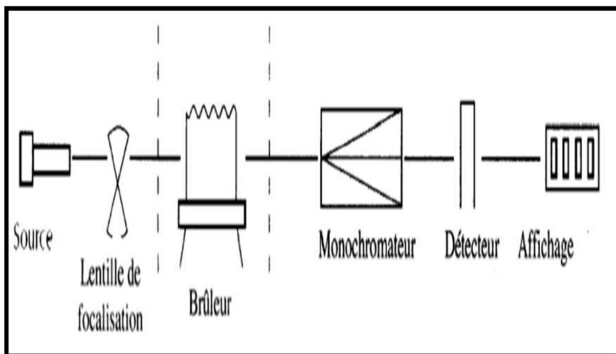
Figure II.12. Schéma de principe fonctionnement de la SAAF.
