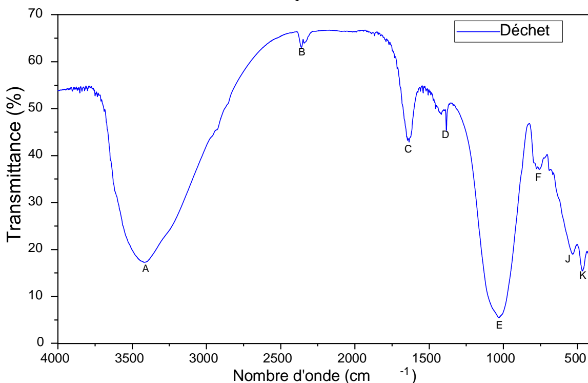
Figure III.2. Spectre infrarouge du déchet de l'unité ENIEM.
