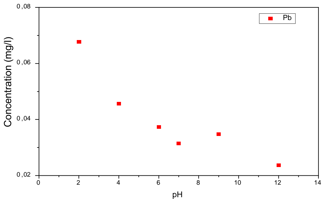
Figure III.6. Evolution de la concentration du plomb en fonction du pH pour le matériau S/S.
