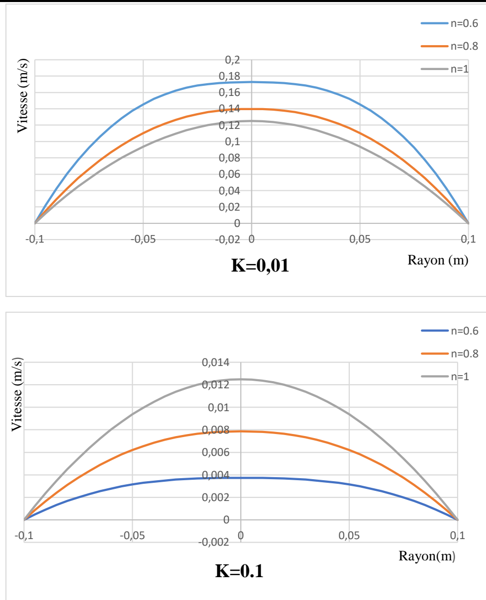
Figure 13: Evolution de vitesse en fonction d'index d'écoulement .
