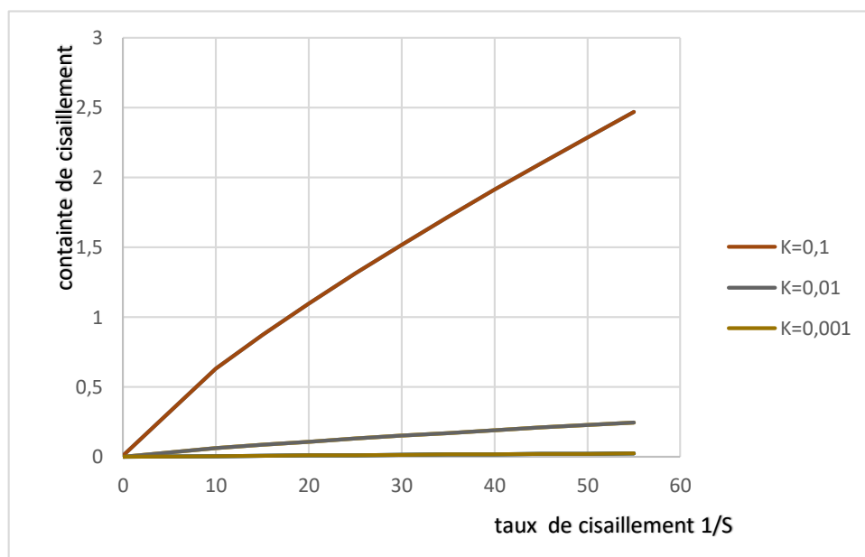
Figure 12: Variation de taux de cisaillement en fonction de la contrainte de cisaillement à différentes viscosités (K).
