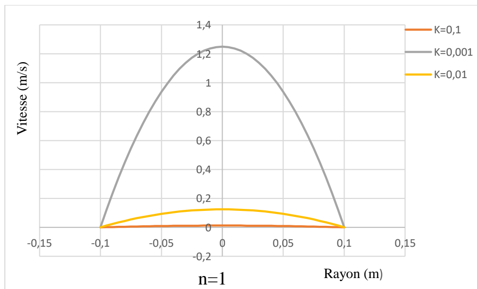
Figure 14: Evolution de la vitesse en fonction du rayon à différentes viscosités.
