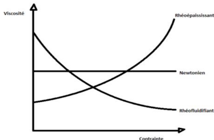
Figure 3: Graphique théorique de la viscosité de plusieurs types de fluides en fonction de la contrainte de cisaillement.
