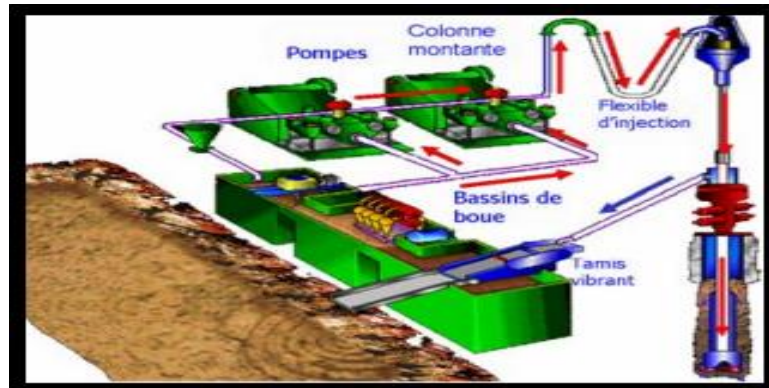
Figure 2: Cycle de fluide sur le site de forage [5]
