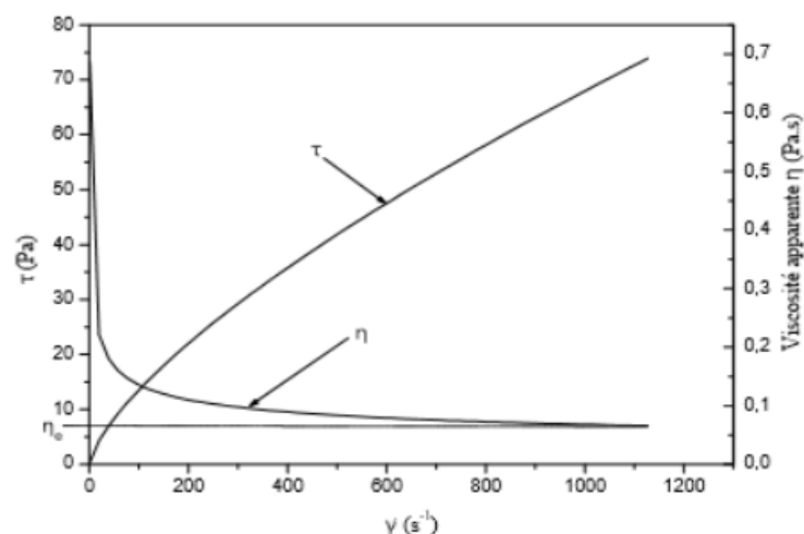
Figure 5: Variation de la contrainte de cisaillement et de la viscosité apparente en fonction de la vitesse de cisaillement pour un fluide rhéofluidifiant.
